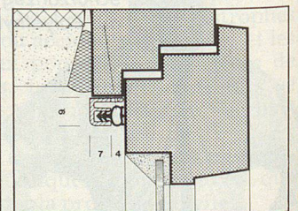
Fenstersanierung HEBGO 121/526
