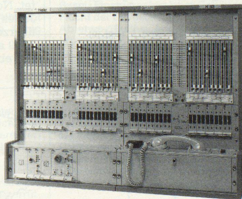
Manuelle Telefonzentrale H 88
