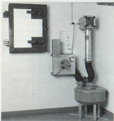
Schutzraum-Abschlüsse und -Belüftungs-Anlagen
