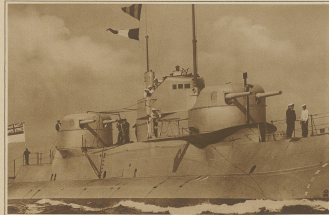
Besser noch keine Abreise. Das neueste englische U-Bootboot, das mit den modernsten Erfindungen der Technik ausgestattet ist.
