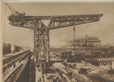
Die größten Drehkräne der Welt befinden sich auf einer Schiffswerft in Hamburg. Der im Bild gezeigte Turm ist gerade in hochgradigem Zustande eine Höhe von über 60 m und ist imstande, 250 Tonnen zu heben
