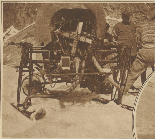
Vorderansicht des Schneemotors. Wie im Bilde ersichtlich ist, werden die Aufpuffgase vorn durch die Schlittkufen abgeleitet. Auf diese Weise kann verhindert werden, daß bei kalter Witterung der Schnee an den Kufen hängen bleibt
