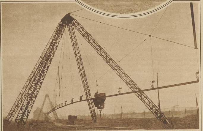
Bei Hamburg ist eine Versuchsbahn zur Beförderung von Lastkähnen erbaut worden. Die Kähne werden durch einen auf einer Schwebeschiene laufenden Motor gezogen
