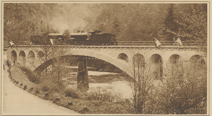
Die im gleichen Stil gehaltene obere Brücke. Durch den großen Bogen ist ein Pfeiler der alten eisernen Brücke sichtbar, die nun abgebrochen wird
