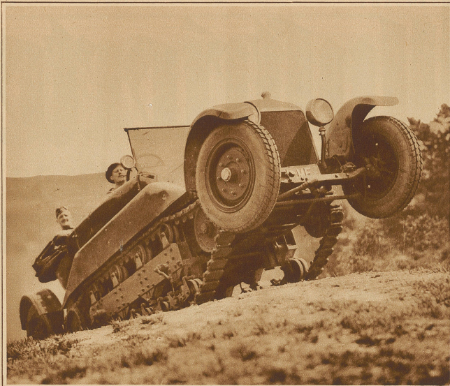
Das neueste Motorfahrzeug stellt eine sinnvolle Kombination von Automobil und Raupenwagen dar. Auf schlechtem Terrain werden die Automoblräder hochgeschaltet. Kehrt das Fahrzeug auf die Straße zurück, so genügt ein Hebelgriff, um es wieder als gewöhnliches Auto fahrbereit zu machen
