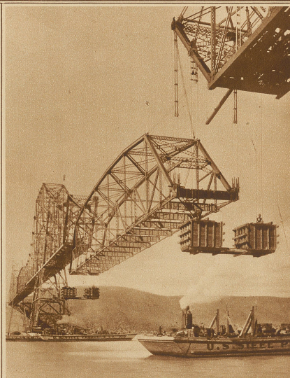
Die Gewalt der Technik. Die neue Eisenbahnbrücke über die Carquinez «Streets» an der San Francisco Bay, die jetzt ihrer Vollendung entgegengeht. Unser Bild zeigt das Einfügen des Mittelstückes überall
