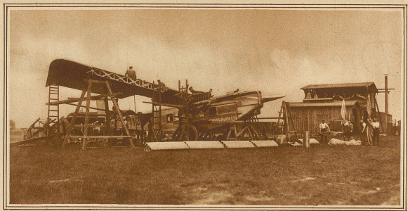
Bau neuer Luftriesen. Montage eines Rohrbach Roland Ganzmetall-Flugzeuges, das nach der Fertigstellung auf der Strecke München-Rom in Verkehr genommen werden soll
