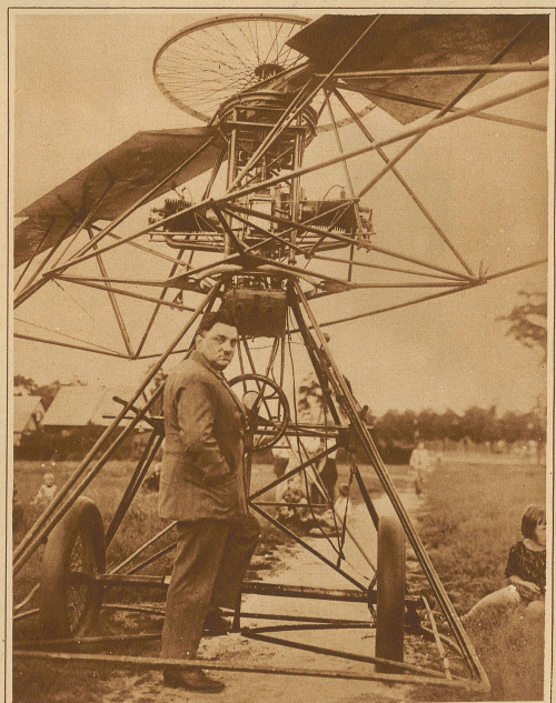
Engelbert Zaschka, ein deutscher Ingenieur, hat ein Hubschraubergezugs konstruiert, das horizontal sein soll, vertikal aufsteigen, in der Luft stillstehen und wieder senkrecht zu landen. Wichtig ist ferner, daß es dem Erfinder geglückt zu sein scheint in der Luft völlige Stabilität und auch ein Gleitvermögen des Flugzeuges zu erreichen. Unser Bild zeigt Ing. Zaschka mit seinem Apparat auf dem Flugplatz Jochensthal
