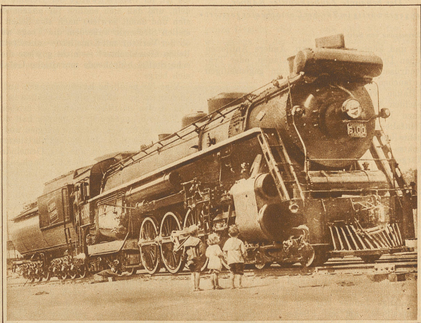
Englands größte Lokomotive, ein Wunder der Technik, ist dieser Tage in den Canadian National Railroad eingeführt worden. Sie entwickelt 3200 P.S.
