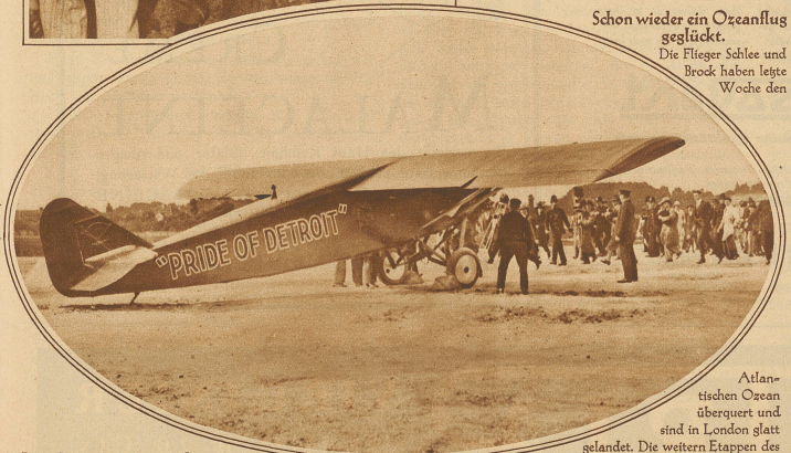
Das Ozeanflugzeug nach seiner Landung auf dem Flugplatz Croyden (London)
