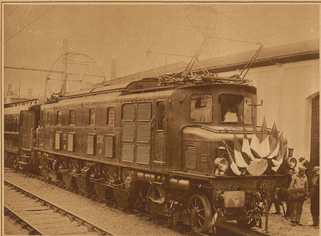
Die elektrische Lokomotive des Einweihungszuges Paris-Vierzon Ein Erfolg schweizerischer elektrischer Lokomotiven in die 204 Kilometer mißt, wurde also in einer Stunde 87 Minuten zurückgelegt, somit ist dies die höchste mittlere Geschwindigkeit, die auf einer längeren Strecke bis jetzt in
