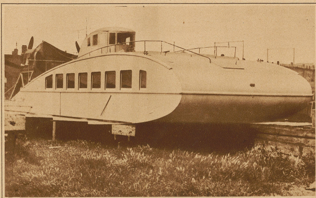
Eine neuartige Schiffs-konstruktion. In Wien wurde kürzlich das erste Gleitboot für den Donauverkehr von Stapel gelassen. Man rechnet allgemein damit, daß dieses eigenartig gebaute Schiffchen gute Dienste leisten wird
