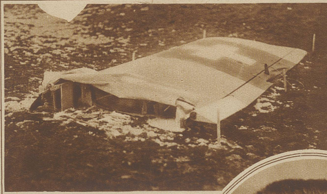
Die während des Fluges gebrochene Tragfläche, die etwa 1 km von der Absturzstelle entfernt gefunden wurde Phot. Jost
