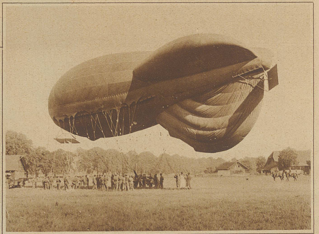
Auch die Schweiz hat ein lenkbares Luftschiff. Der in Italien gekaufte Fesselballon ist mit einem Motor ausgerüstet worden. Die ersten, in Bern vorgenommenen Flugversuche, ergaben befriedigende Resultate Phot. Kettel
