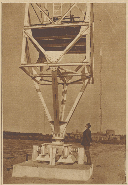
Der größte Rundfunksender Europas ist dieser Tage in Zeesen (Deutschland) eröffnet worden. Unser Bild zeigt das untere Ende eines der beiden 210 m hohen Masten, die nur auf einer kleinen Stahlkugel von 9 cm Durchmesser ruhen
