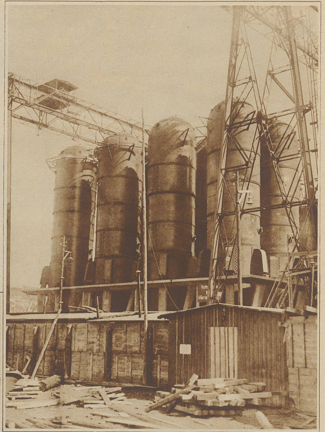
Eine riesige Dampfspeicheranlage ist vom Charlottenburger Elektrizitätswerk errichtet worden. Jeder Kessel ist 23 Meter hoch und hat 4,5 Meter Durchmesser. In diesen Riesentuben wird der am Tage nicht benötigte Dampf aufgespeichert, mit dem dann am Abend noch weitere 40 000 Kilowattstunden Strom erzeugt werden können
