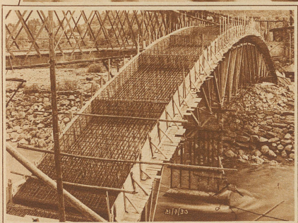
Die neue Brücke kurz vor dem Einsturz. Der flache Bogen hat eine Stützweite von 88 m. Der Gerüstpfiler in der Mitte ist dann zusammengebrochen
