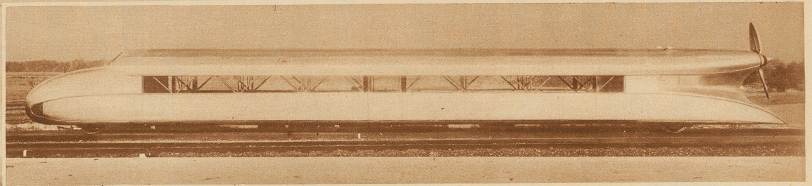
Der neue Propeller-Triebwagen von der Seite gesehen. Bei einer Länge von 26 Meter bietet er Platz für 40 Personen
