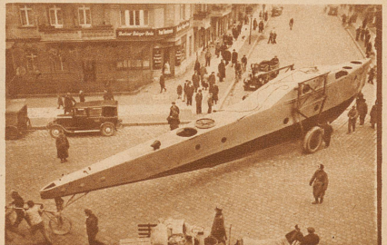
Ein Ungeheuer in Berlin. Der Rumpf des Flugbootes «Rohrbach-Romar» in den Straßen Berlins auf dem Transport nach Frankreich, für das es gebaut wurde
